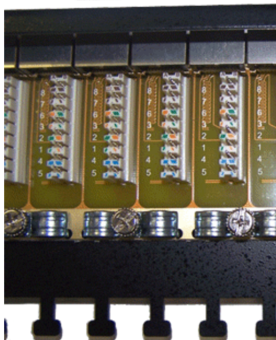
Крепежные винты
