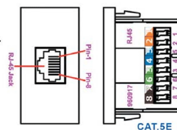
Цоколевка
