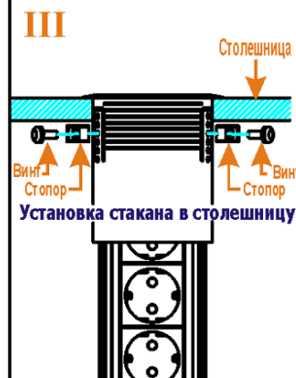
Диаметр установочного отверстия 82 мм
