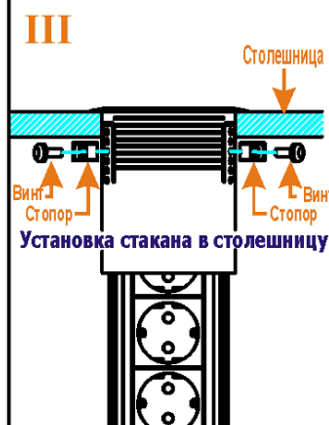
Диаметр установочного отверстия 82 мм
