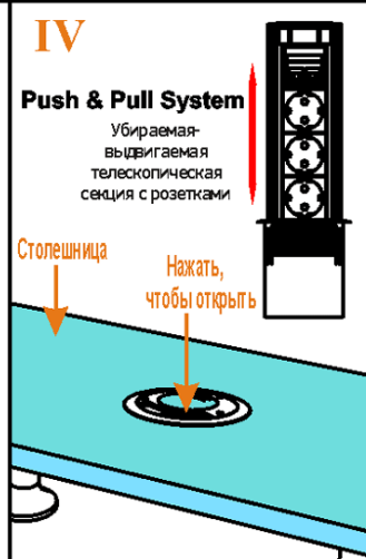
Миниколонна монтируется в отверстие
