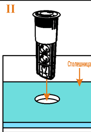
Миниколонна монтируется в отверстие
