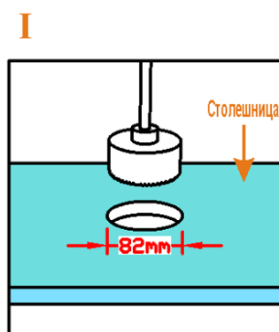
Диаметр установочного отверстия 82 мм
