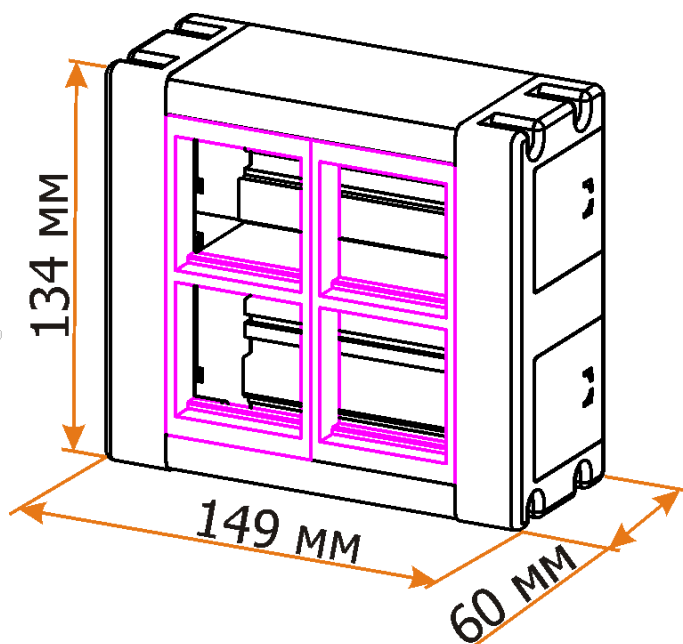
Размеры
