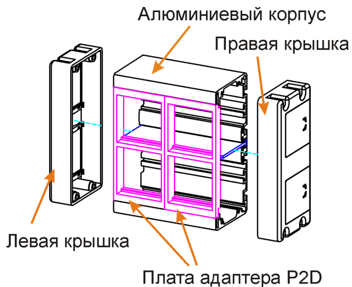
Конструкция
