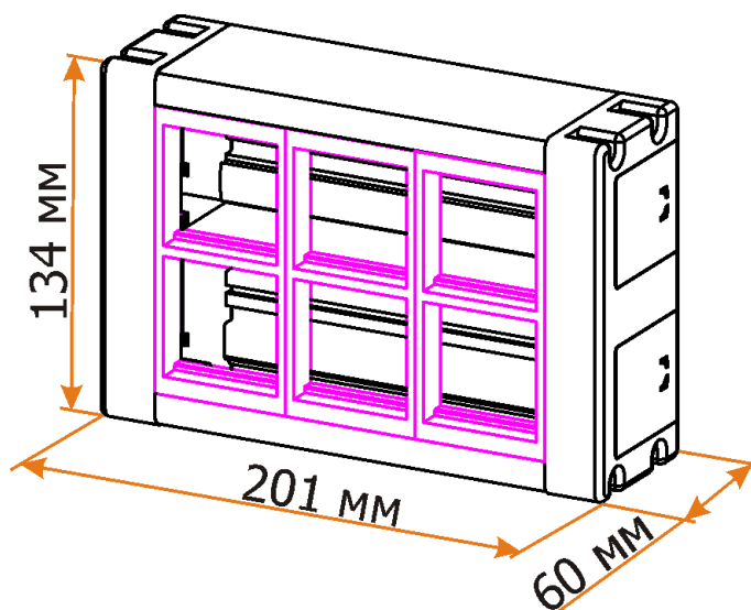
Размеры
