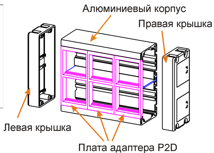
Конструкция
