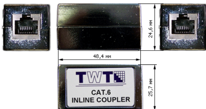
Размеры повторителя
