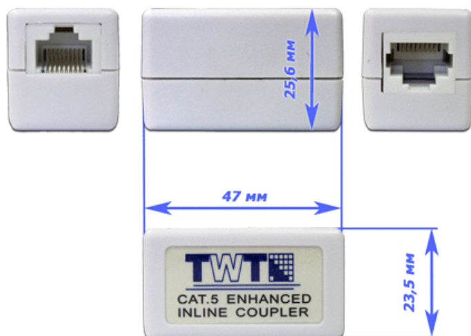
Размеры повторителя
