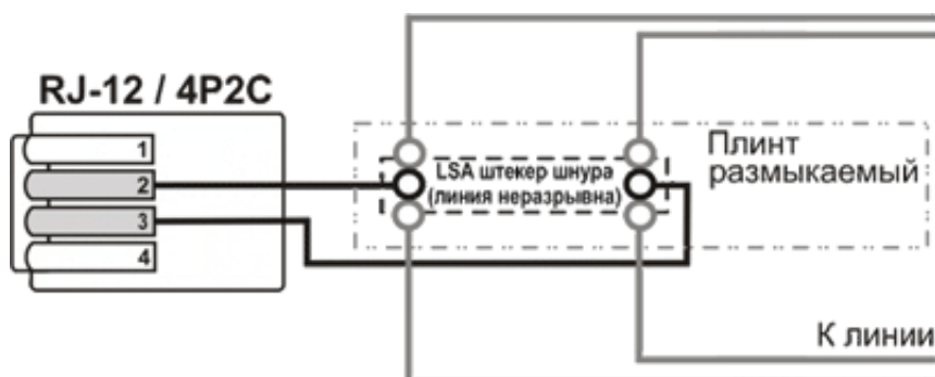
Схема подключения шнура
