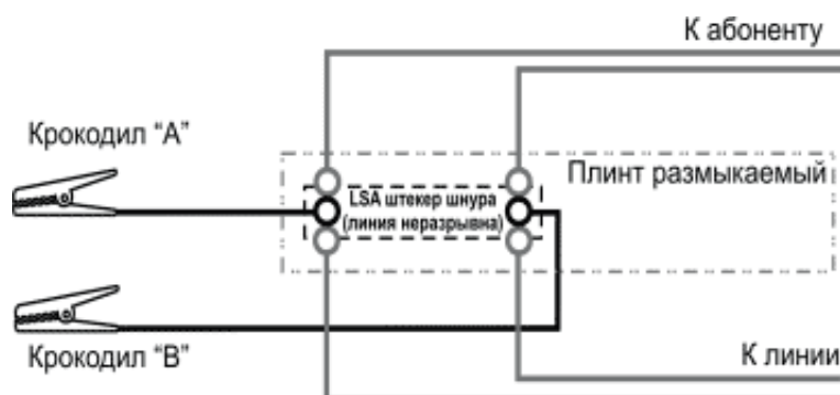
Схема подключения шнура
