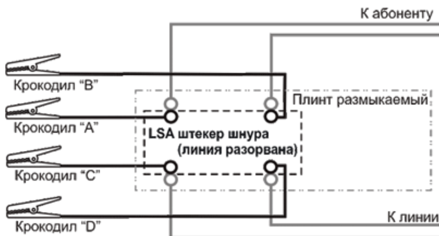
Схема подключения шнура
